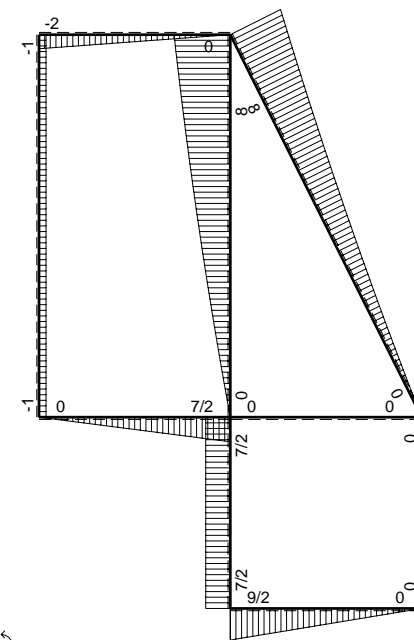
\oplus M 0 flessione da carichi assegnati
